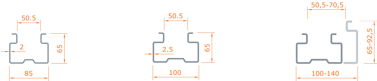
Typ RS13-85-65
